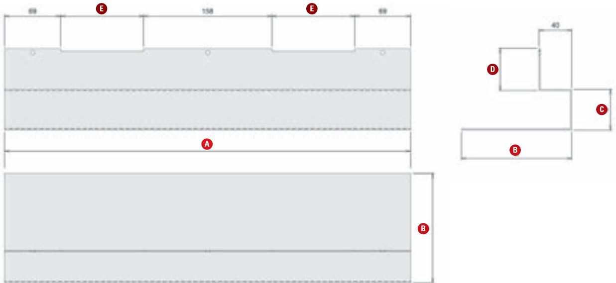
Profil départ type N°1
