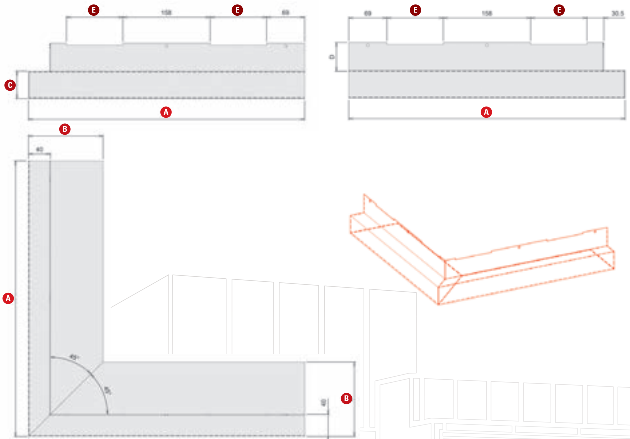
Profil départ d'angle
